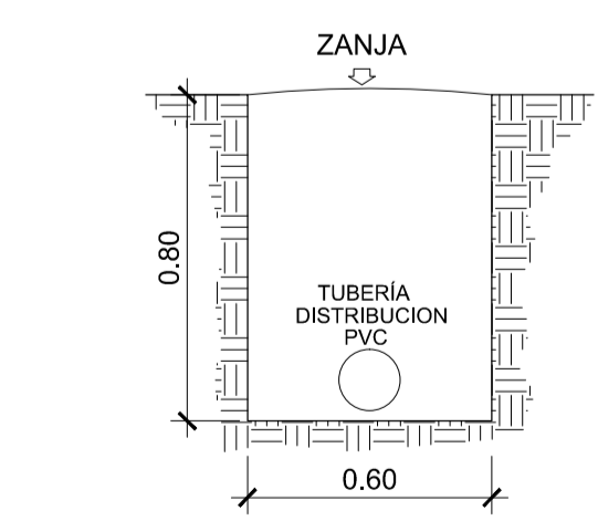
DETALLE DE ZANJA DISTRIBUCION ESCALA: 1:20
