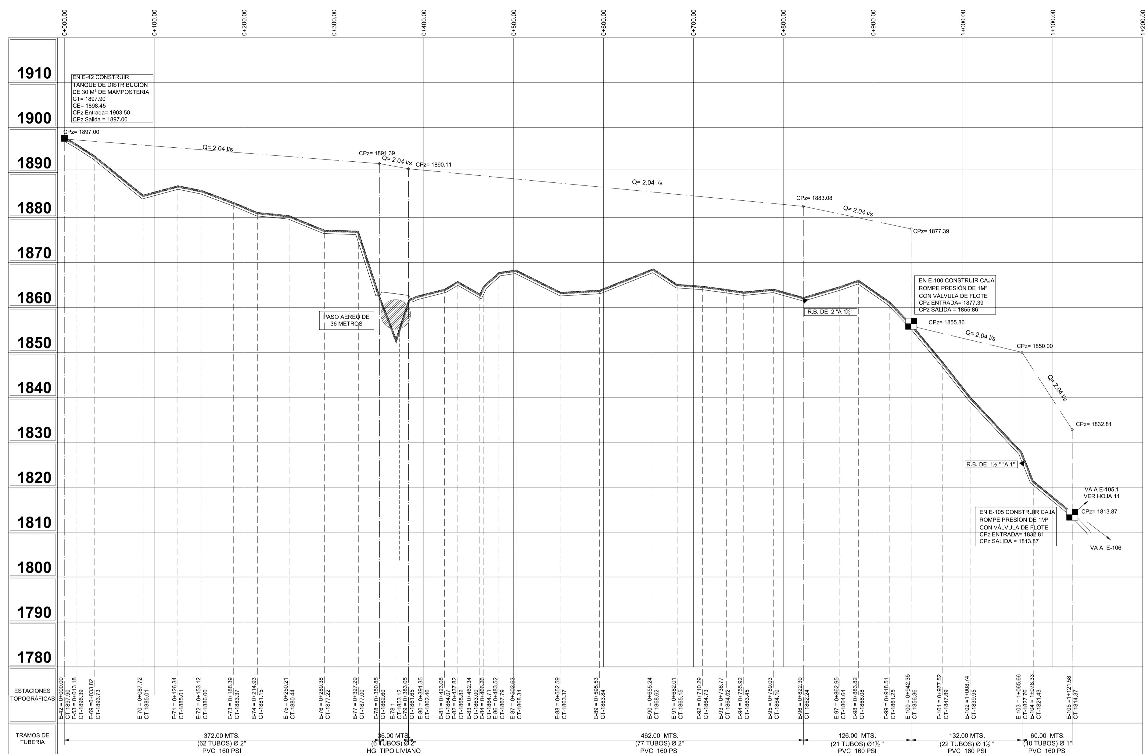
PERFIL RAMAL 3.0 DE E-42 T.D. A E-105 C.R.P. +V.F. ESCALA HORIZONTAL: 1:2500 ESCALA VERTICAL: 1:500
