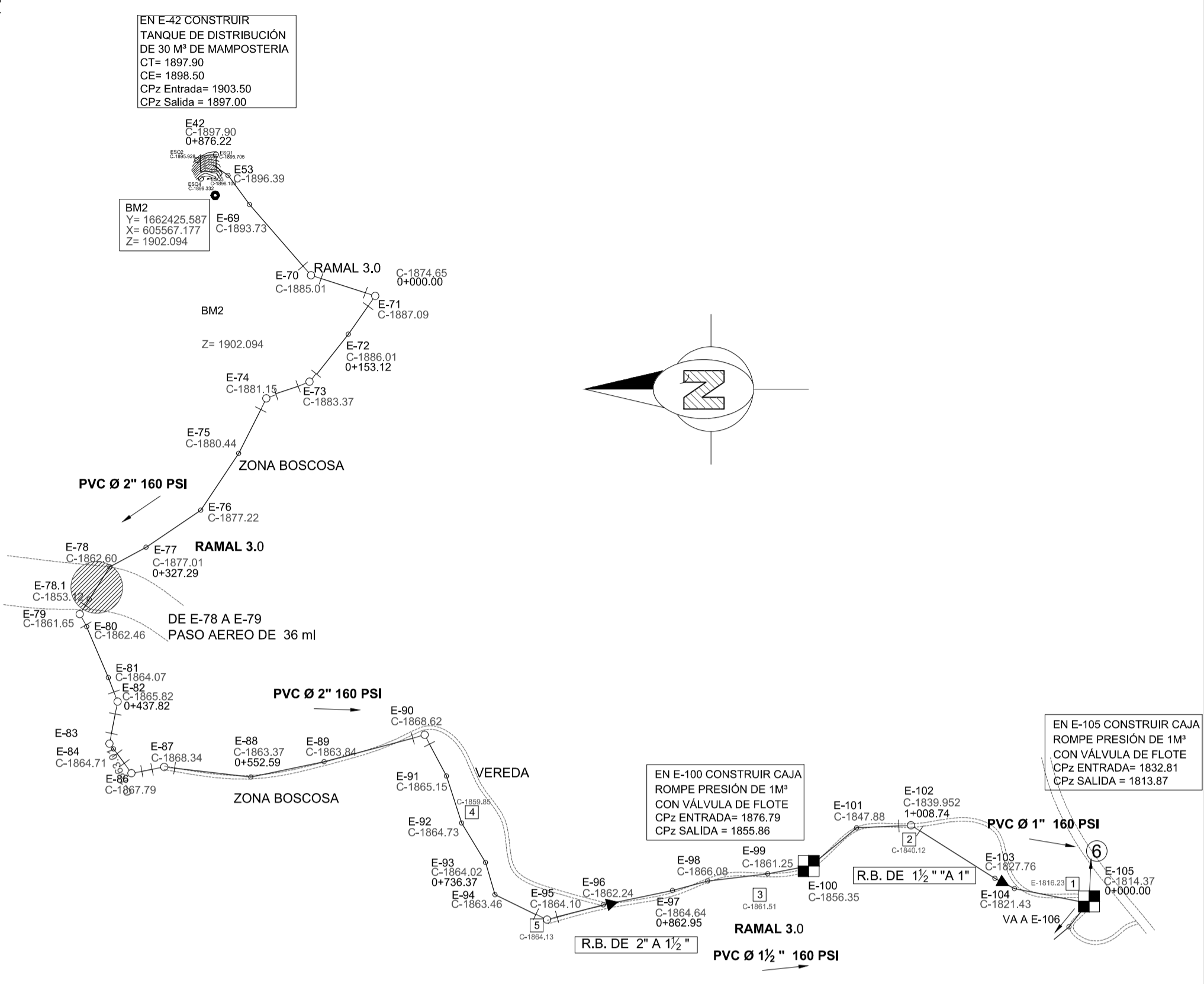
PLANTA RAMAL 3.0 DE E-42 T.D. A E-105 C.R.P. +V.F. ESCALA: 1:500
