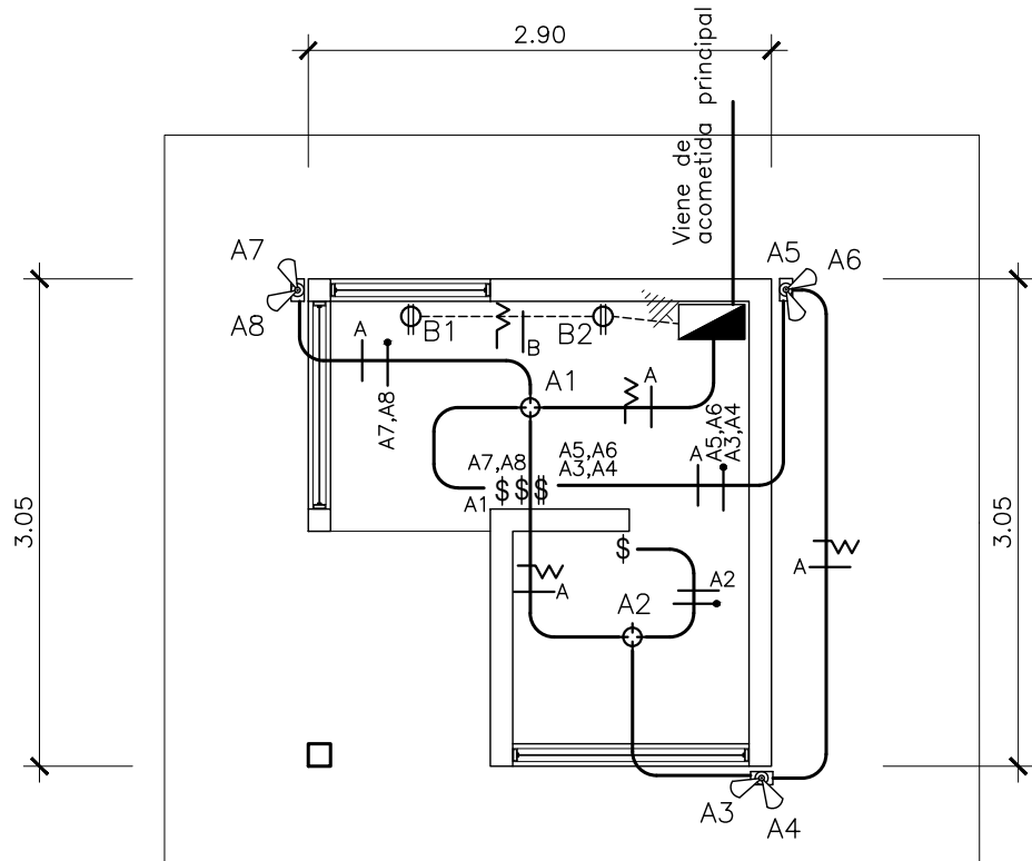
PLANTA BAJA INSTALACION ELECTRICA -ILUMINACION Y FUERZA-
