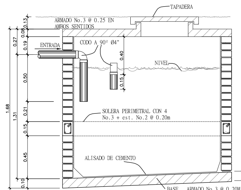
SECCION FOSA SEPTICA ESC. 1/50
