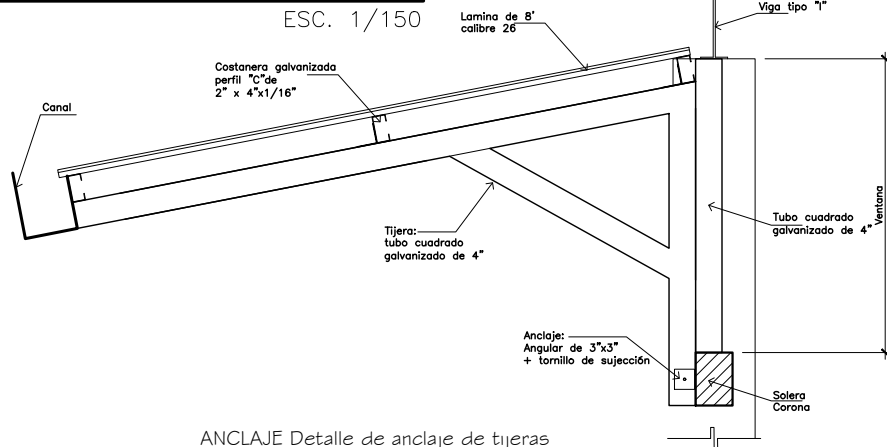
ANCLAJE Detalle de anclaje de tijeras en Ventanas
