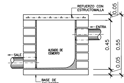
CORTE A-A DETALLE DE CAJA DE REGISTRO AGUA PLUVIAL
