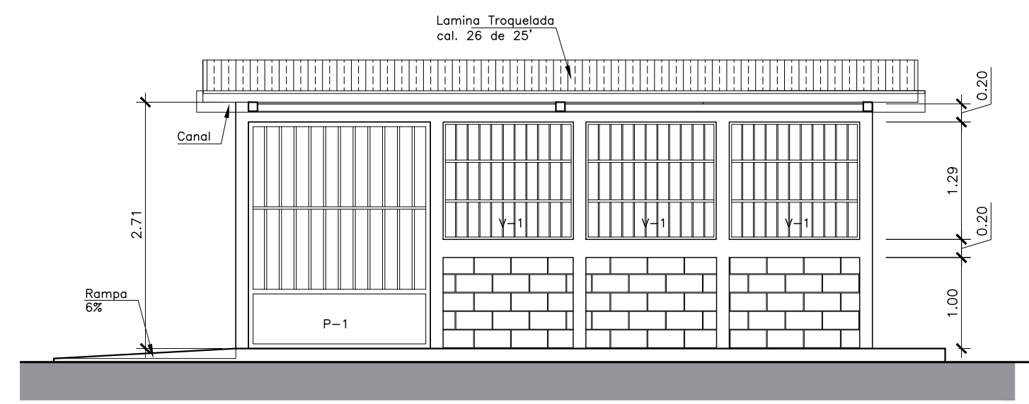
ELEVACION NORTE BODEGA ESC. 1/50
