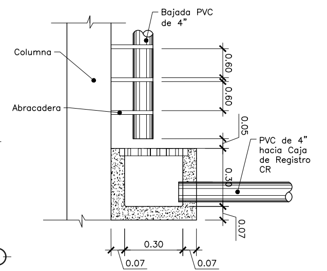
DETALLE DE CAJA RECOLECTORA AGUA PLUVIAL
