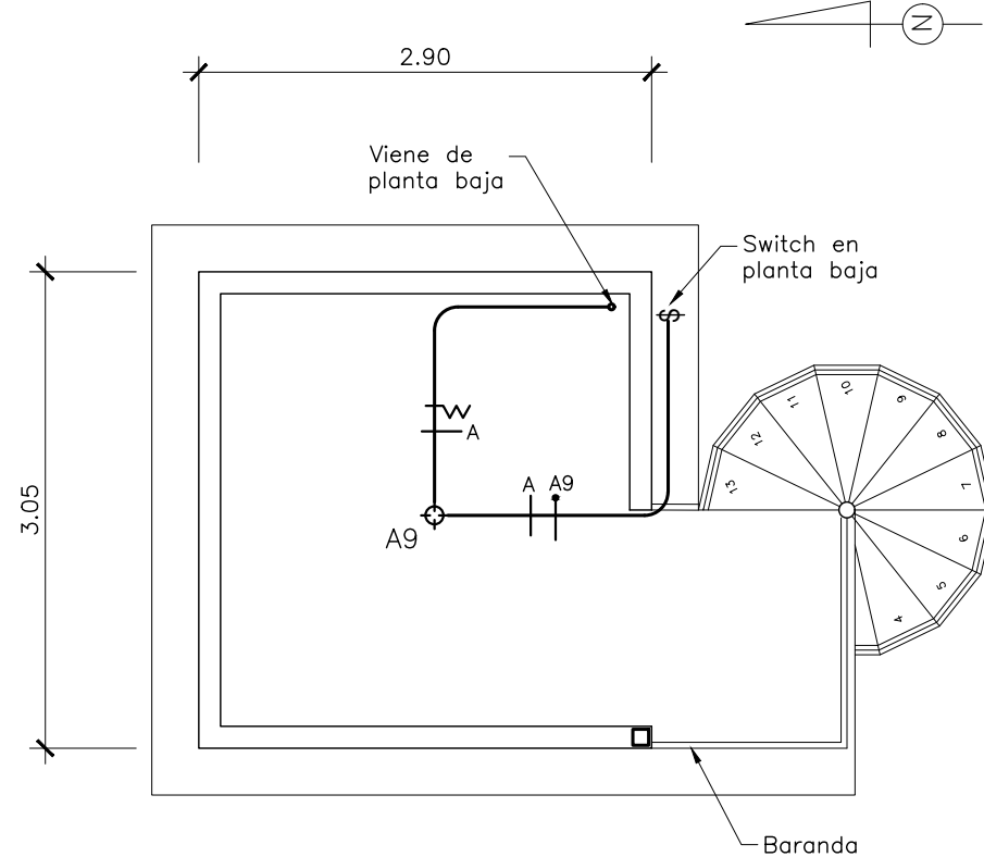
PLANTA ALTA INSTALACION ELECTRICA -ILUMINACION Y FUERZA-
