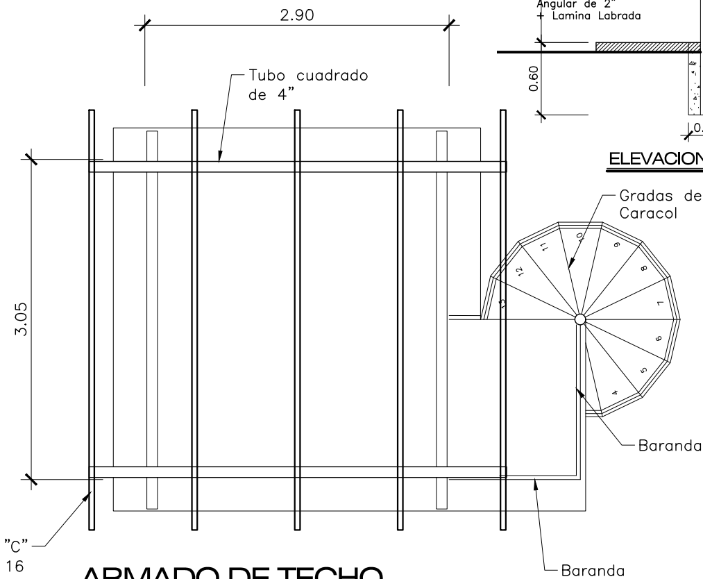
ARMADO DE TECHO
