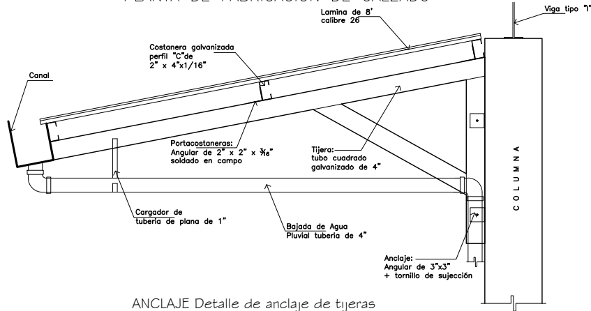
ANCLAJE Detalle de anclaje de tijeras en Columnas
