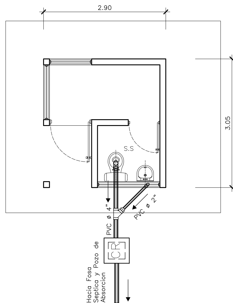
PLANTA INSTALACION SANITARIA -DRENAJE- ESC. 1/50
