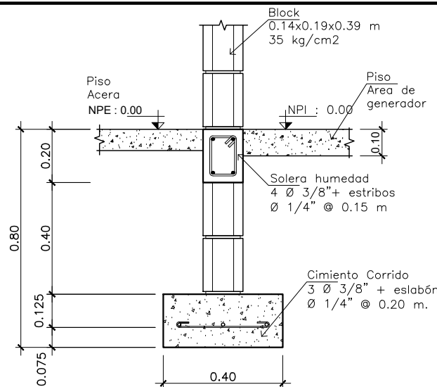
CIMIENTO CORRIDO CC-1 ESC: 1:20
