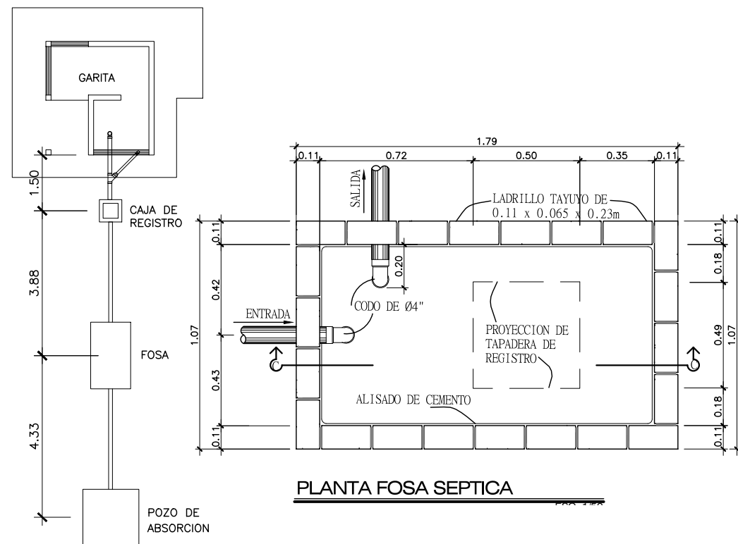
Ubicacion Instalaciones Drenaje GARITA ESC. 1/125
