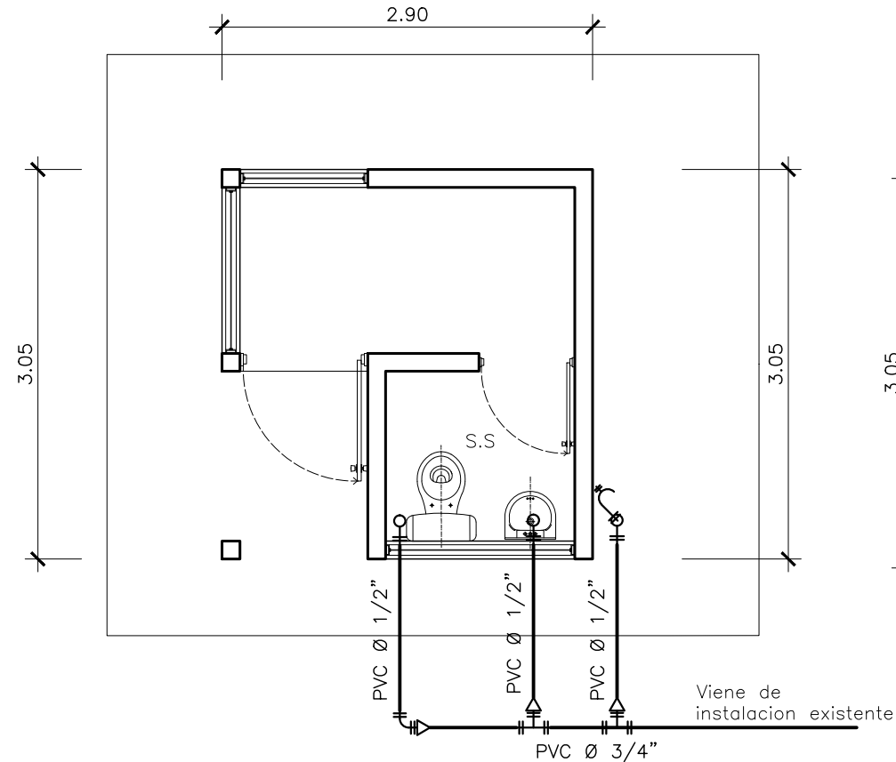
PLANTA INSTALACION HIDRAULICA -AGUA POTABLE- ESC. 1/50
