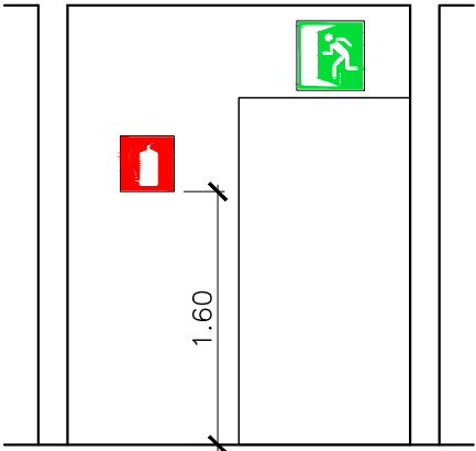
DETALLE DE COLOCACION DE ROTULO EN MURO
