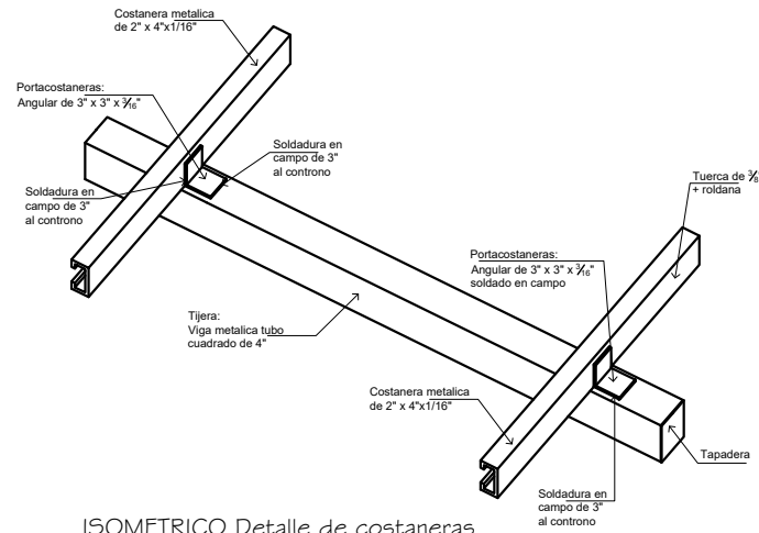
ISOMETRICO Detalle de costaneras
