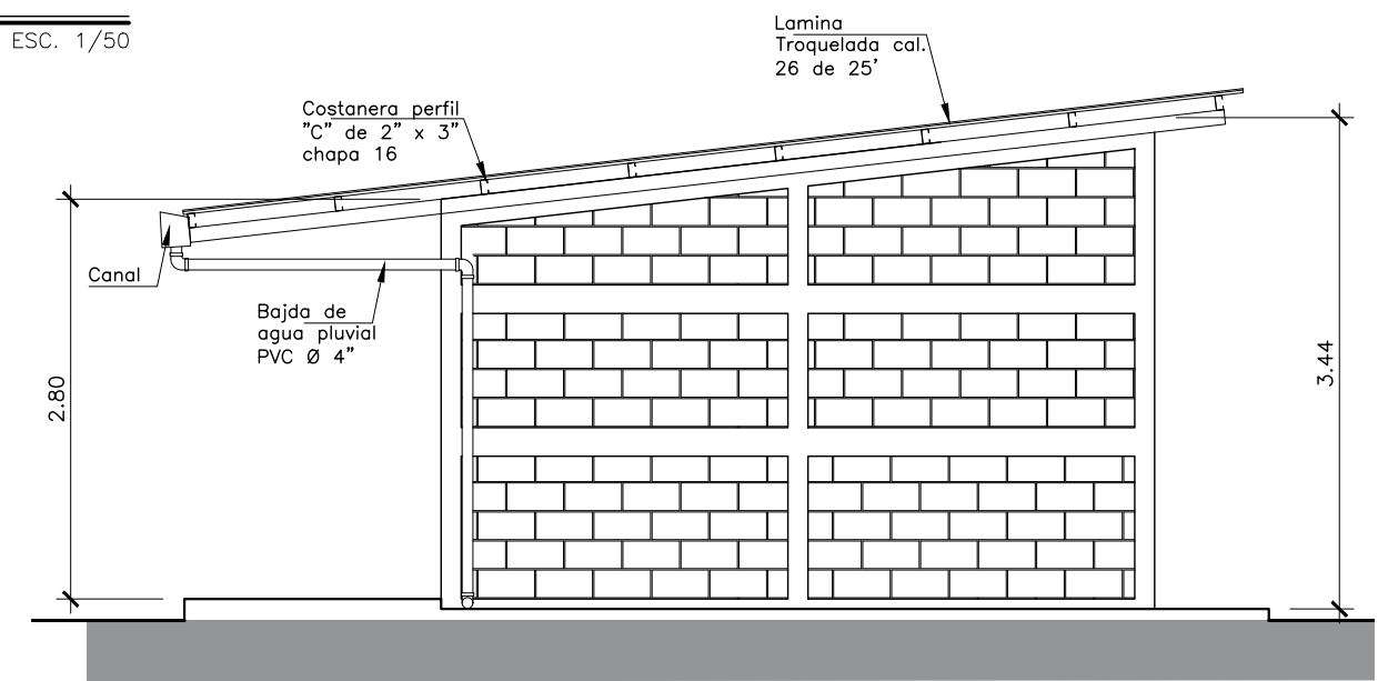
ELEVACION OESTE BODEGA ESC. 1/50
